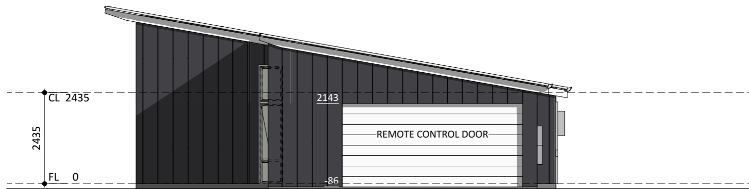
ELEVATION 4 1:100
