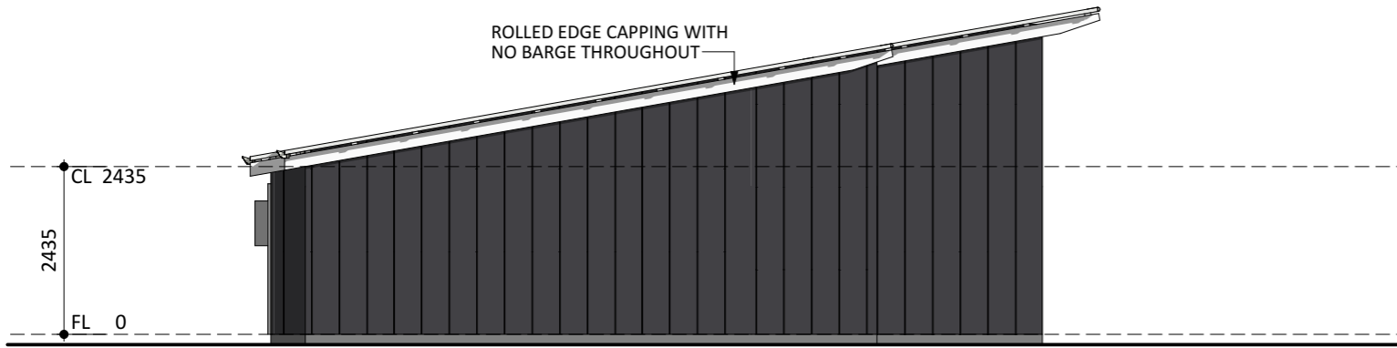
ELEVATION 2 1:100
